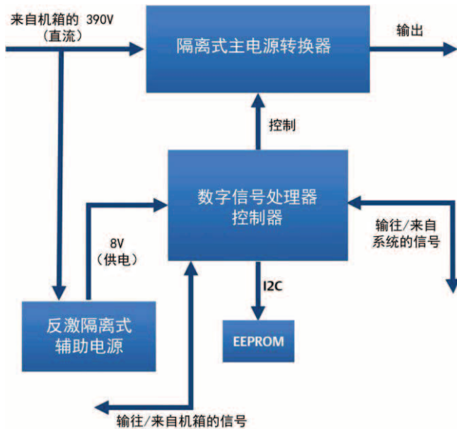
内置于可配置电源之内并可利用数字信号处理器进行控制的典型输出模块 - 结构框图
